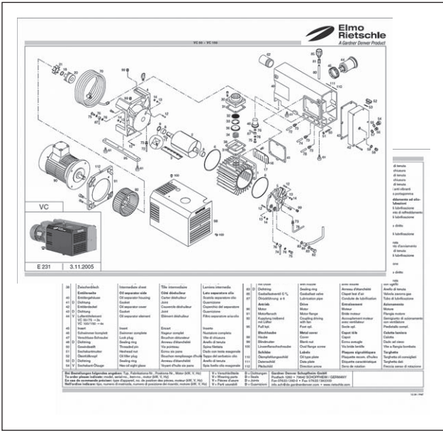
Fig. 13 Elenco parti di ricambio (esempio)
