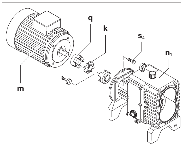
Fig. 10 Giunto C-VLR 60
