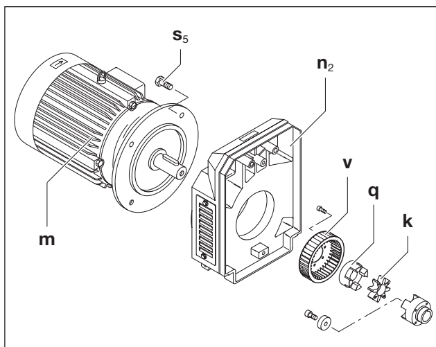
Fig. 11 Giunto C-VLR 100 - 500
